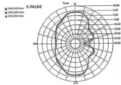
2.4GHz E-Plane
